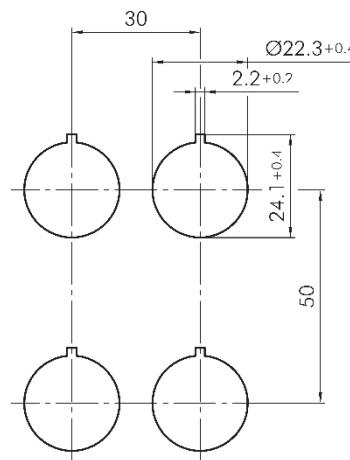
Bohrbild
