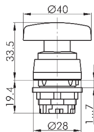
Maßskizze
