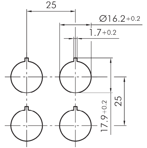
Bohrbild
