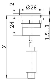
Maßskizze
