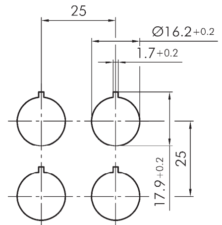
Bohrbild
