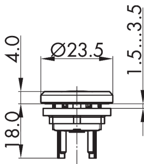
Maßskizze
