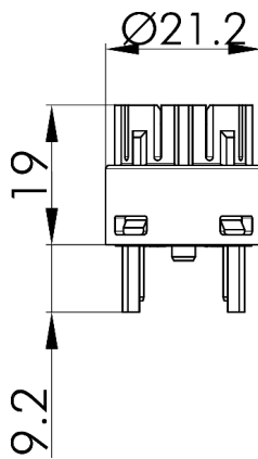
Maßskizze
