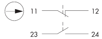
Schaltbild
