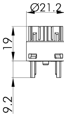
Maßskizze
