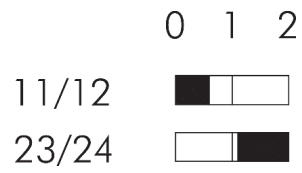
Schaltwegdiagramm
