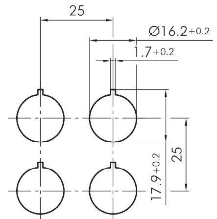
Bohrbild
