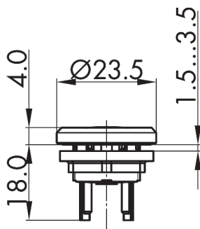
Maßskizze
