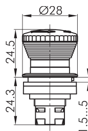
Maßskizze
