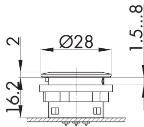
Maßskizze
