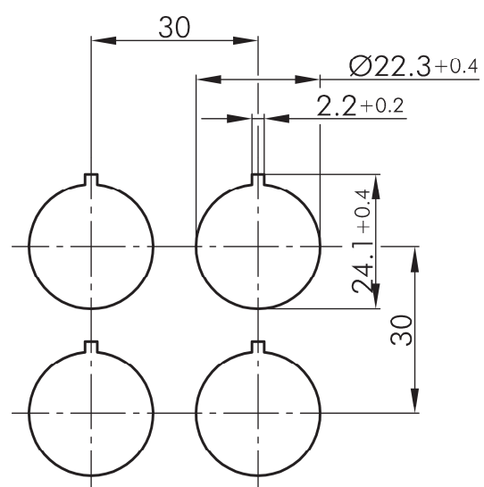
Bohrbild
