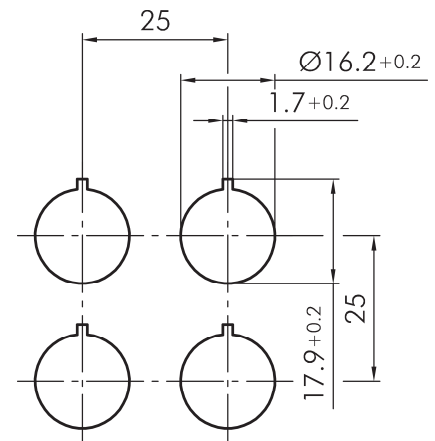
Bohrbild
