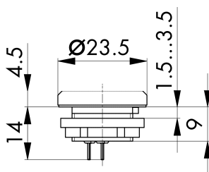
Maßskizze
