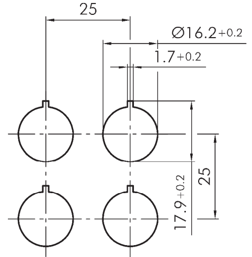
Bohrbild
