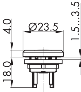
Maßskizze
