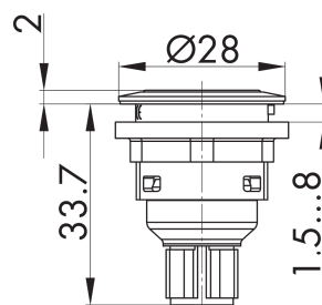
Maßskizze
