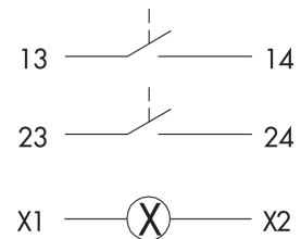
Schaltbild
