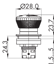
Maßskizze
