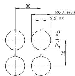
Bohrbild
