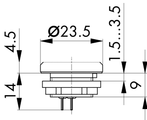
Maßskizze
