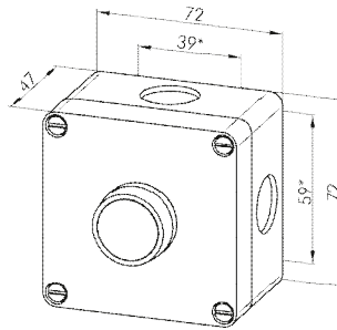
Maßskizze
