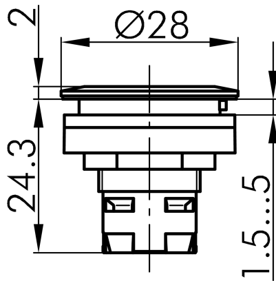
→ Massskizze
