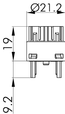
Maßskizze
