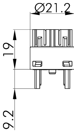
Maßskizze
