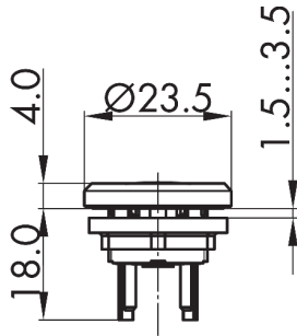
Maßskizze
