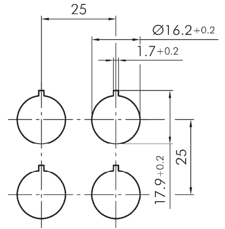
Bohrbild
