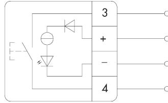
Schaltbild
