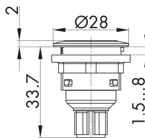
Maßskizze
