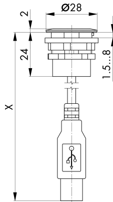
→ Massskizze
