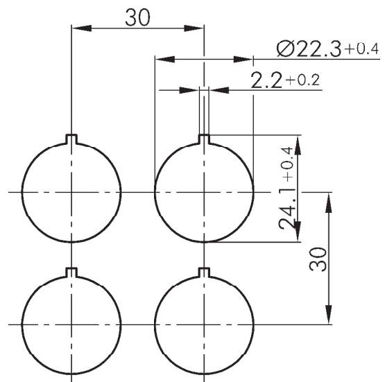
Bohrbild
