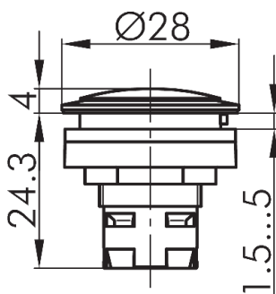
Maßskizze
