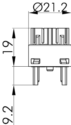
Maßskizze
