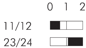
Schaltwegdiagramm
