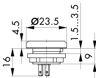
Maßskizze
