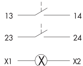
Schaltbild
