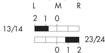
Schaltwegdiagramm
