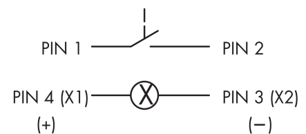
Schaltbild
