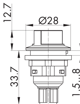
Maßskizze
