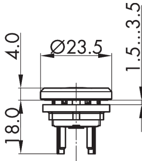
Maßskizze
