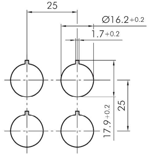
Bohrbild
