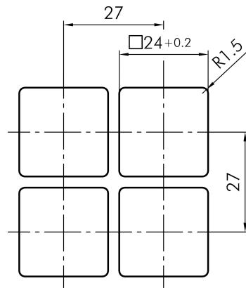
→ Bohrbild
