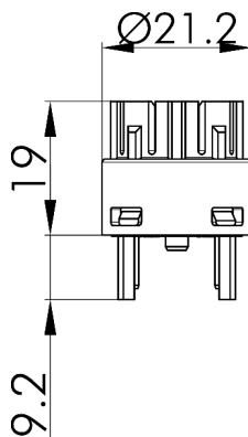
Maßskizze
