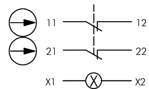
Schaltbild
