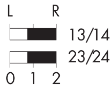
Schaltwegdiagramm
