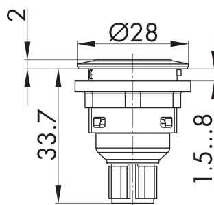
Maßskizze
