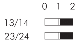
Schaltwegdiagramm
