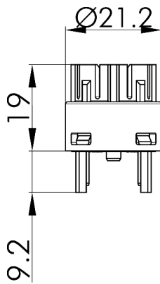
Maßskizze
