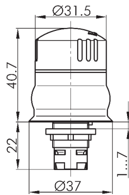
Maßskizze
