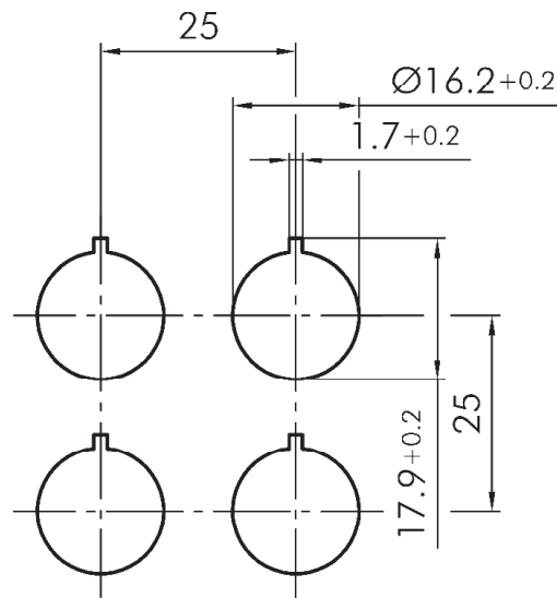
Bohrbild
