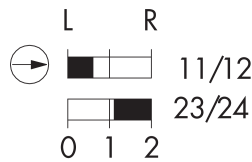
Schaltwegdiagramm
