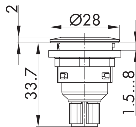
Maßskizze
