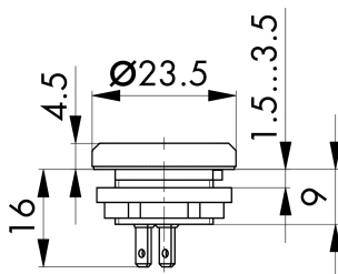
Maßskizze
