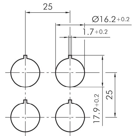
Bohrbild
