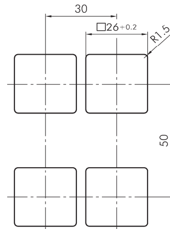
Bohrbild
