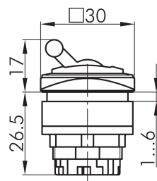
Maßskizze
