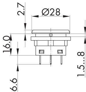
Maßskizze
