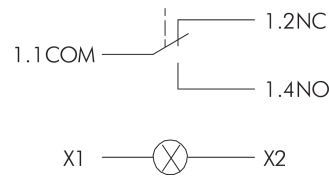
Schaltbild
