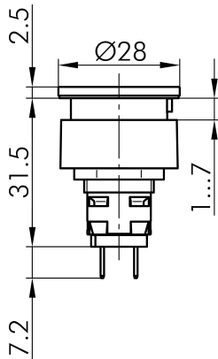
→ Massskizze
