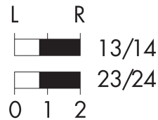
Schaltwegdiagramm
