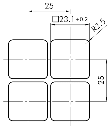
→ Bohrbild
