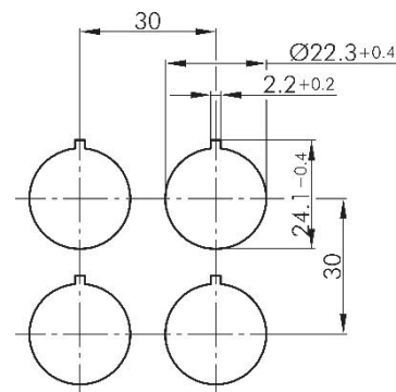
Bohrbild
