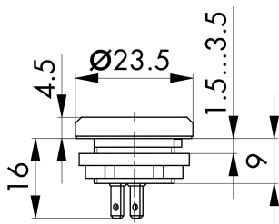
Maßskizze
