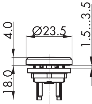
Maßskizze
