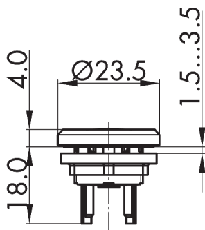
Maßskizze
