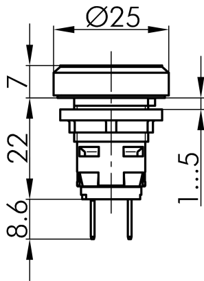
→ Massskizze
