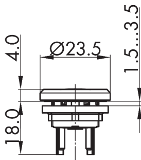
Maßskizze
