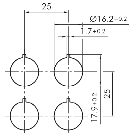
Bohrbild
