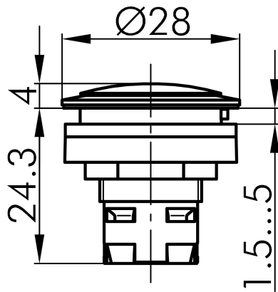
→ Massskizze
