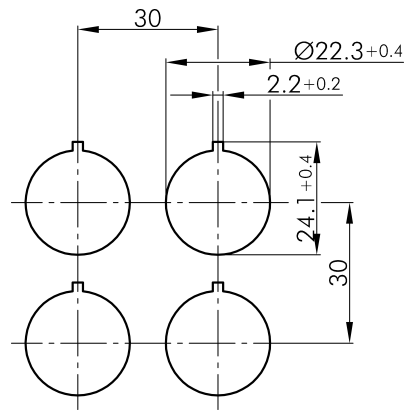
→ Bohrbild
